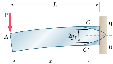
Fig. 6.35 ( PL > M_Y )
