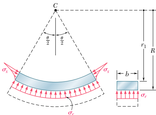
Fig. P4.191
