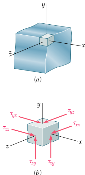
Fig. 3.43 Corner element.
