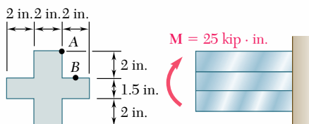
Fig. P4.1
