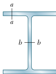
W8 \times 31
