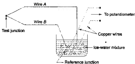
Fig. 2.4 Thermocouple
